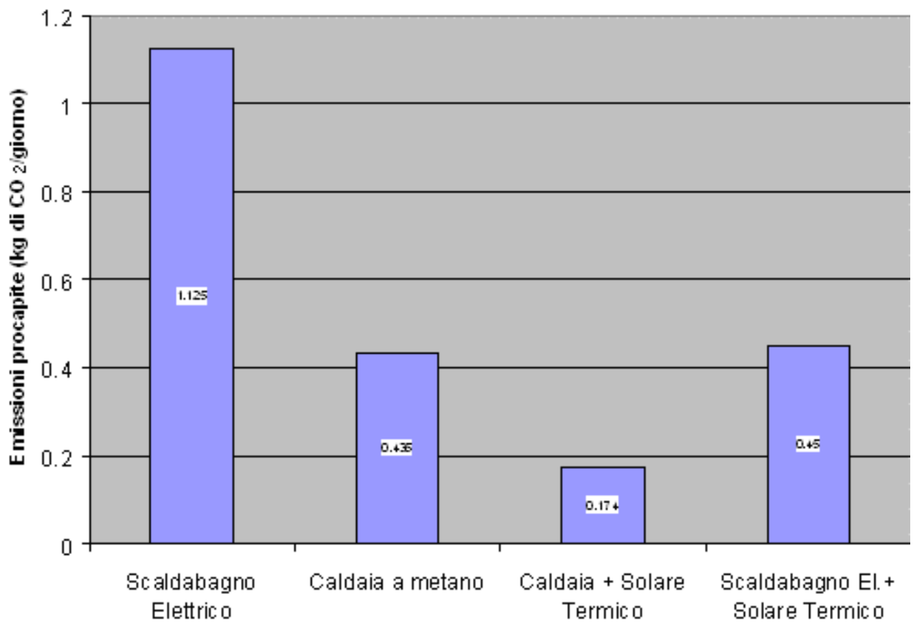
Confronto sulle emissioni di anidride carbonica causate dalle diverse soluzioni esaminate
